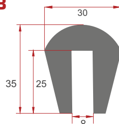
Защитный профиль PG8 на плоскую сталь 8 мм
