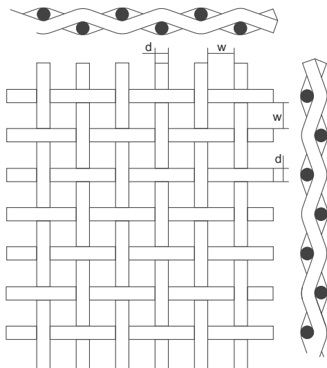
Рисунок 1. Прямое переплетение
