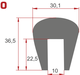
Защитный профиль PG10
