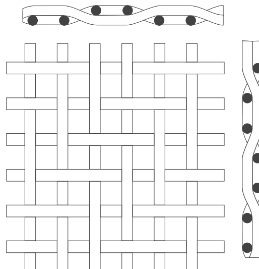
Рисунок 2. Саржевое переплетение
